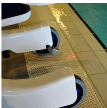
Système de détection infrarouge du bord du bassin avec alarme sonore (option)
